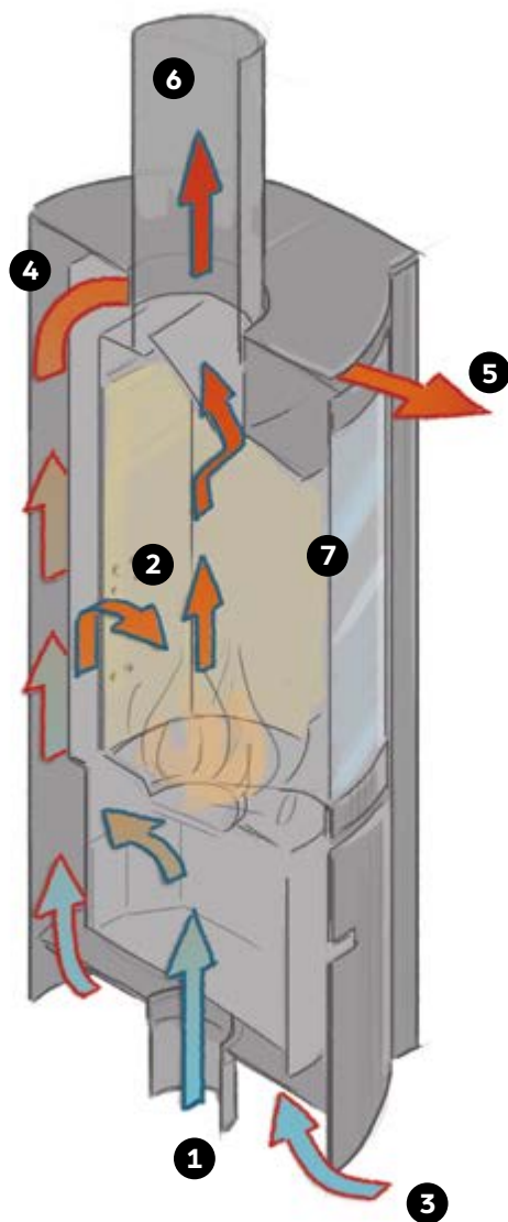
Technique de combustion et circulation de l'air Stûv 30-compact
