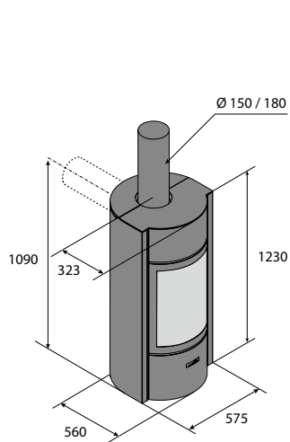
Stûv 30
